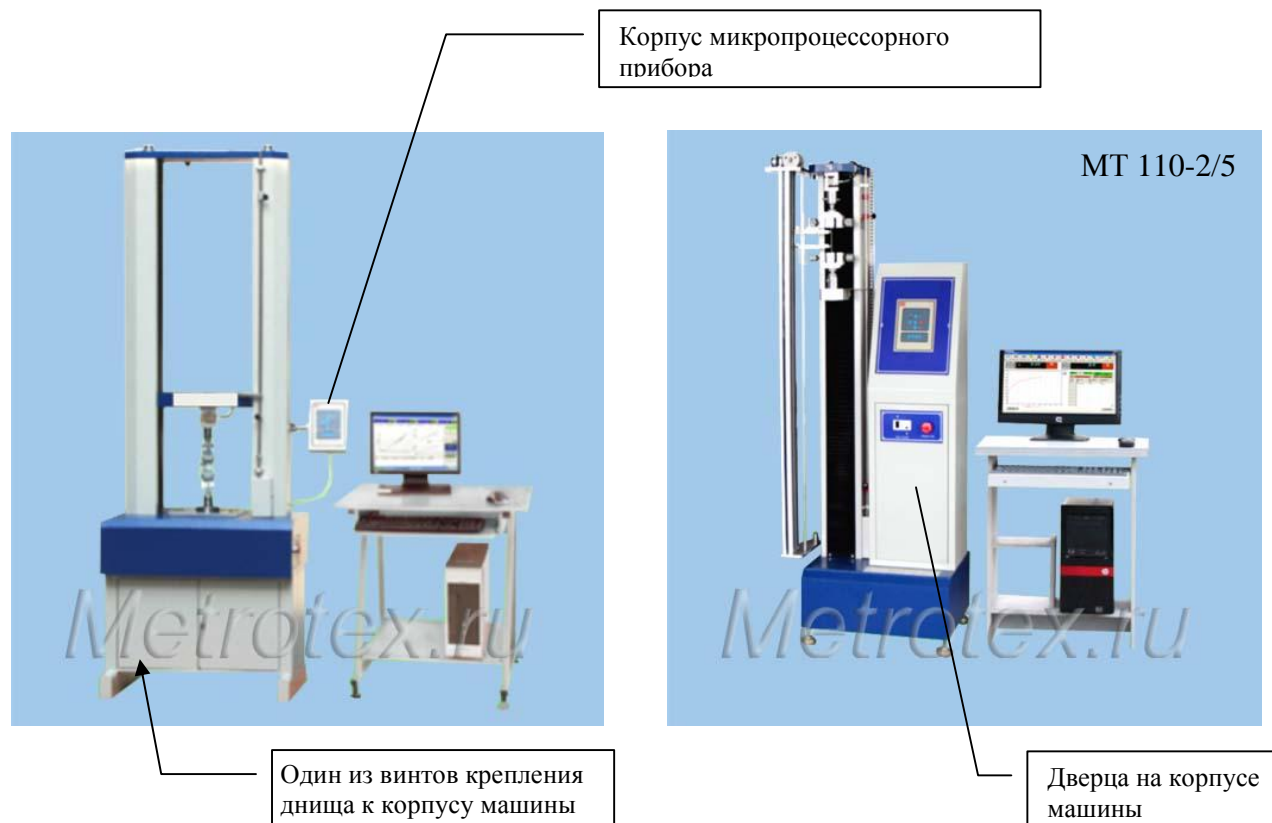
Рисунок 5 – Схема пломбировки машины
